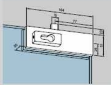
Beispiel Universal-Eckschloss für Glasausschnitt
