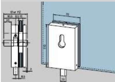
Beispiel Eckschloss
